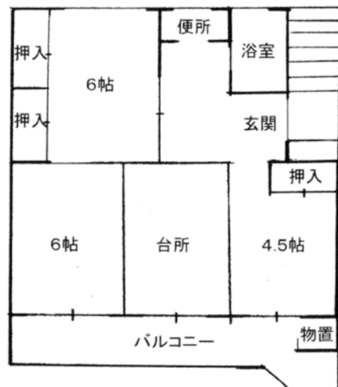
平面図
