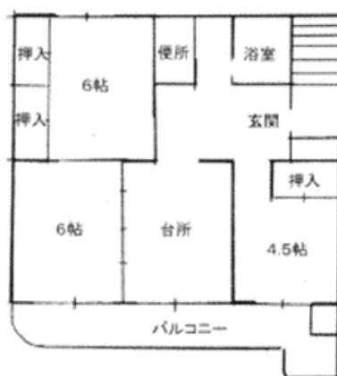
1・2号棟平面図
